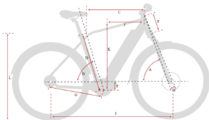
Abbildung S1: Masszeichnung PowerDrive. Die beiden Rahmenarten / Varianten unterscheiden sich nur durch die Form des Oberrohrs / 28 Zoll Radgrösse
